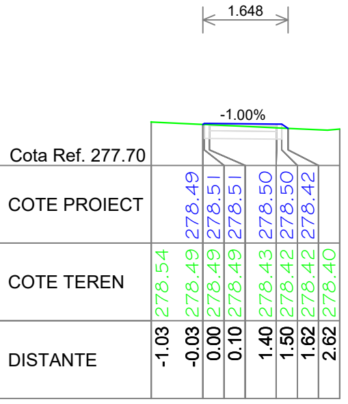
Pz. KM 875.00 Trotuar proiectat
