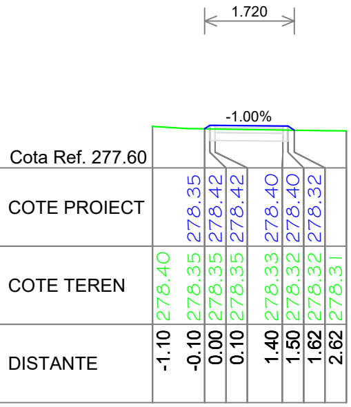
Pz. KM 900.00 Trotuar proiectat
