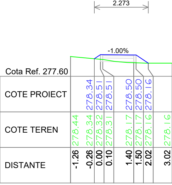
Pz. KM 850.00 Trotuar proiectat
