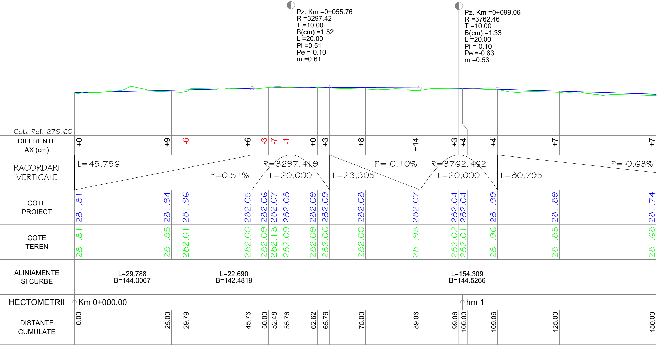
PROFIL LONGITUDINAL Trotuar proiectat DE LA 0.000 LA 150.000 SCARA : ORIZ 1 :500 VERT 1 :100
