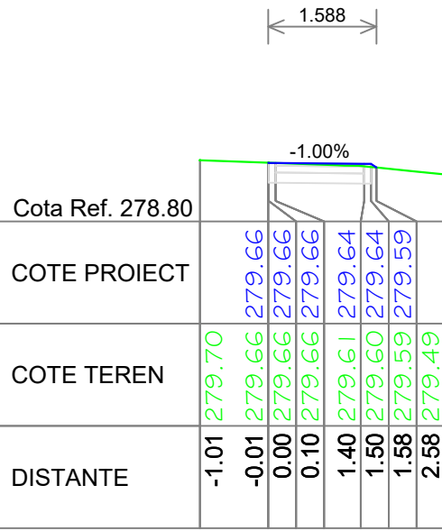
Pz. KM 625.00 Trotuar proiectat
