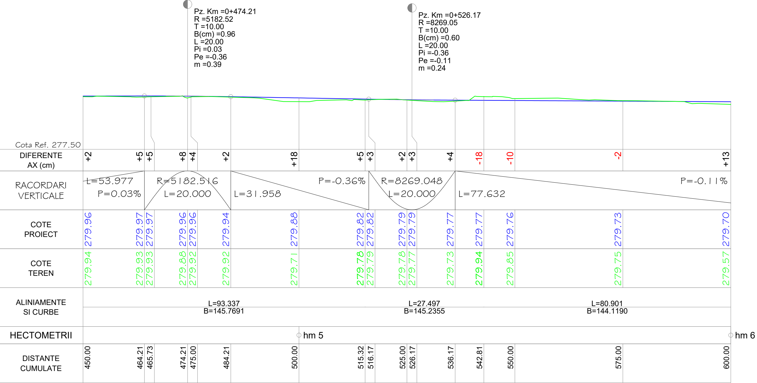
PROFIL LONGITUDINAL Trotuar proiectat DE LA 450.000 LA 600.000 SCARA : ORIZ 1 :500 VERT 1 :100
