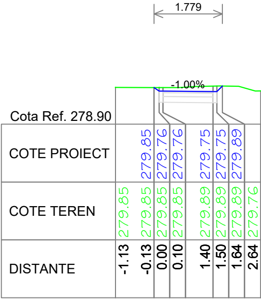
Pz. KM 550.00 Trotuar proiectat
