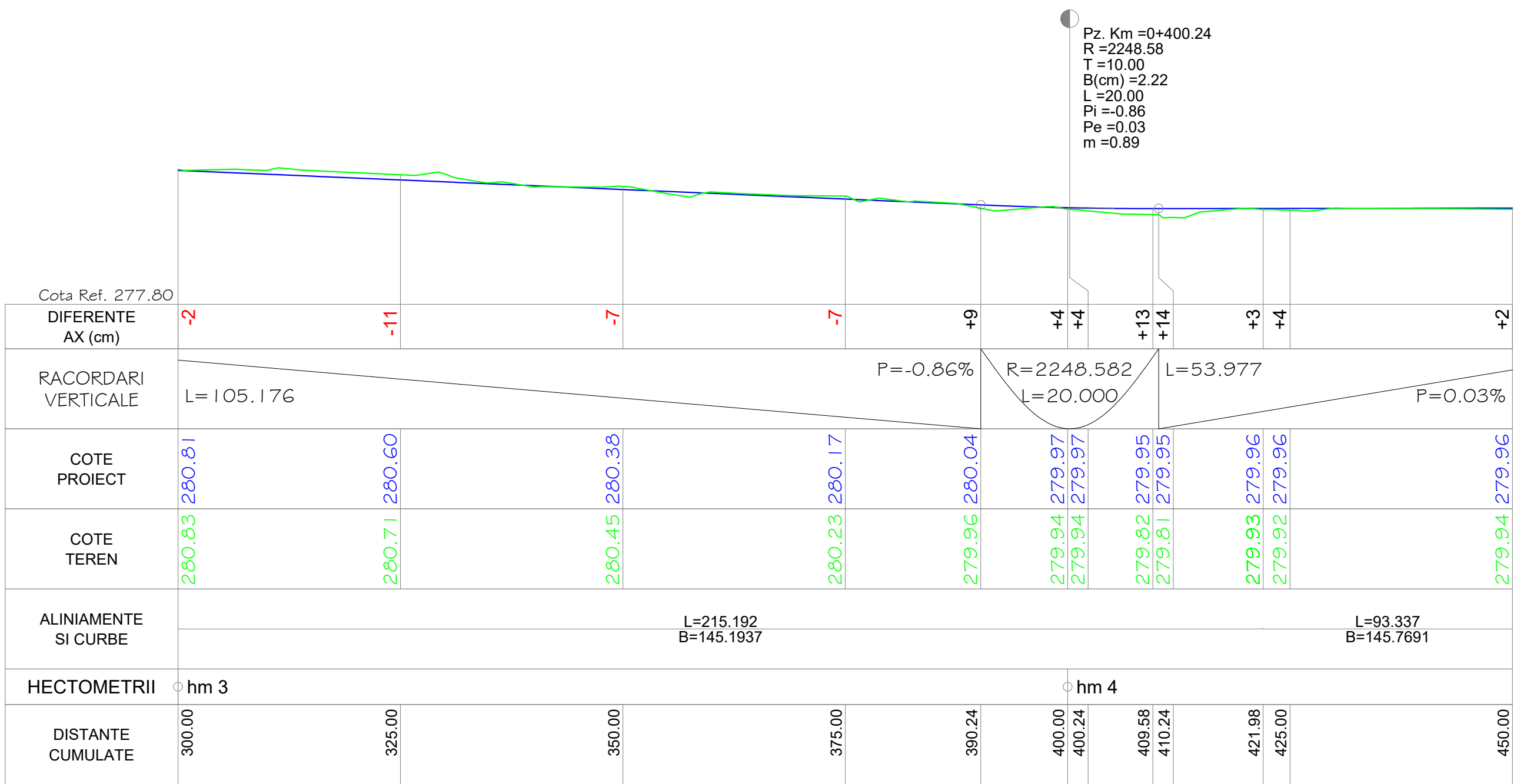
PROFIL LONGITUDINAL Trotuar proiectat DE LA 300.000 LA 450.000 SCARA : ORIZ 1 :500 VERT 1 :100
