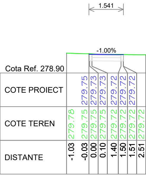
Pz. KM 575.00 Trotuar proiectat
