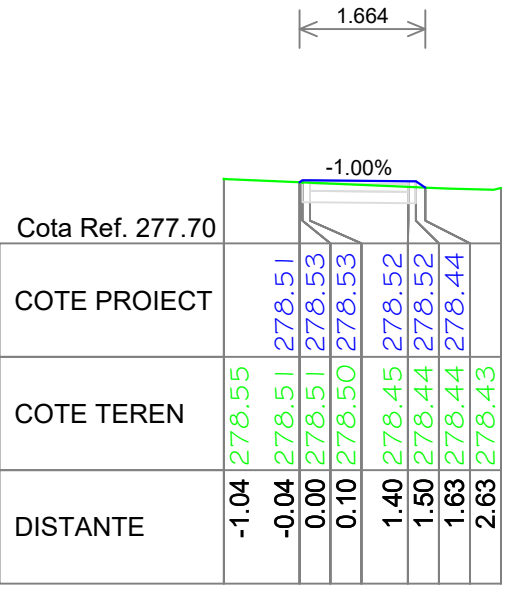
Pz. KM 800.00 Trotuar proiectat
