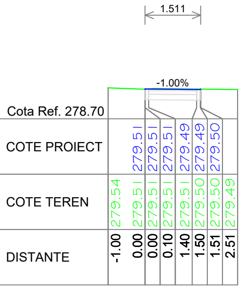
Pz. KM 650.00 Trotuar proiectat
