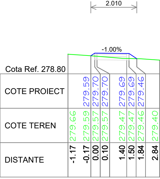
Pz. KM 600.00 Trotuar proiectat
