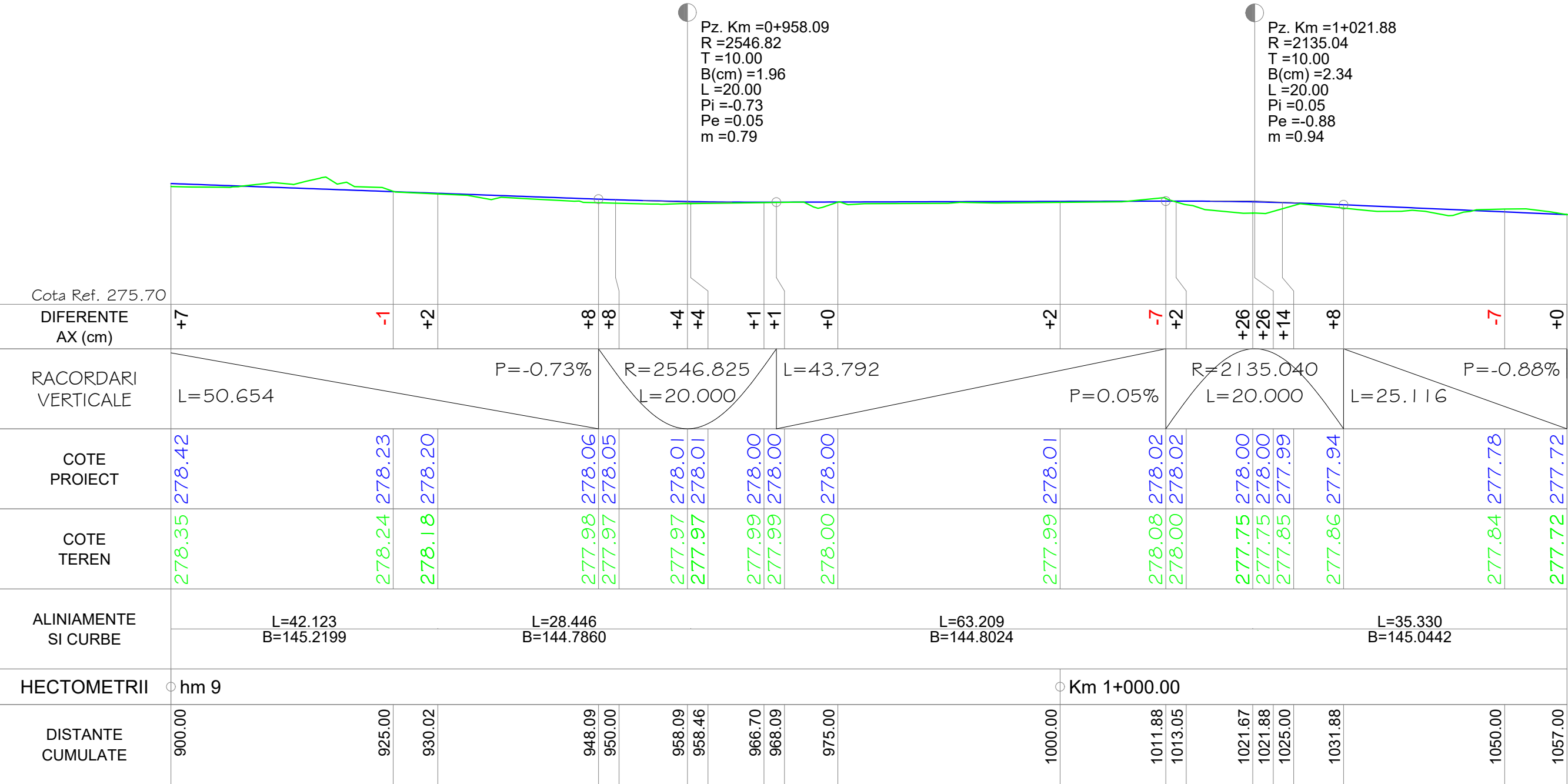
PROFIL LONGITUDINAL Trotuar proiectat DE LA 900.000 LA 1057.000 SCARA : ORIZ 1 :500 VERT 1 :100
