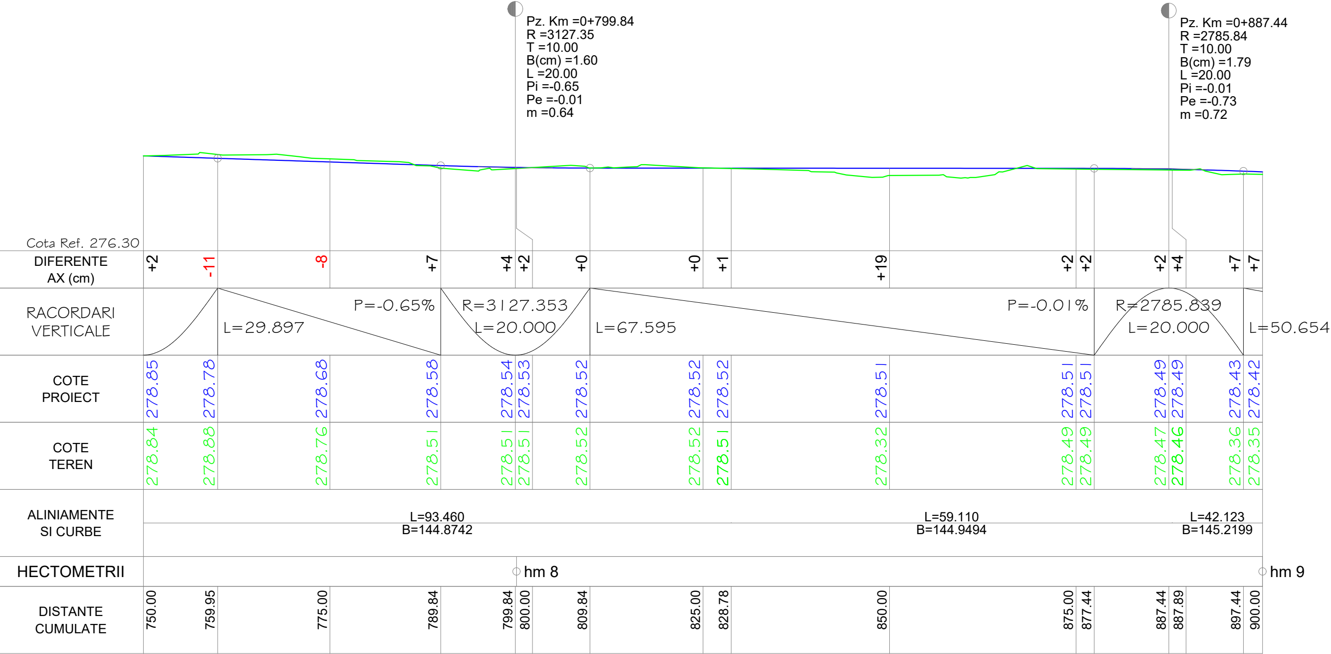
PROFIL LONGITUDINAL Trotuar proiectat DE LA 750.000 LA 900.000 SCARA : ORIZ 1 :500 VERT 1 :100
