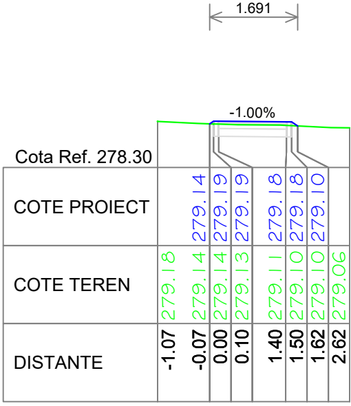
Pz. KM 700.00 Trotuar proiectat
