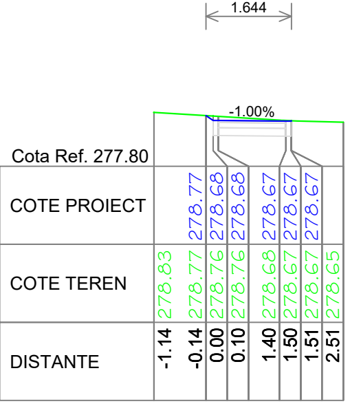
Pz. KM 775.00 Trotuar proiectat
