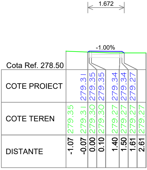
Pz. KM 675.00 Trotuar proiectat
