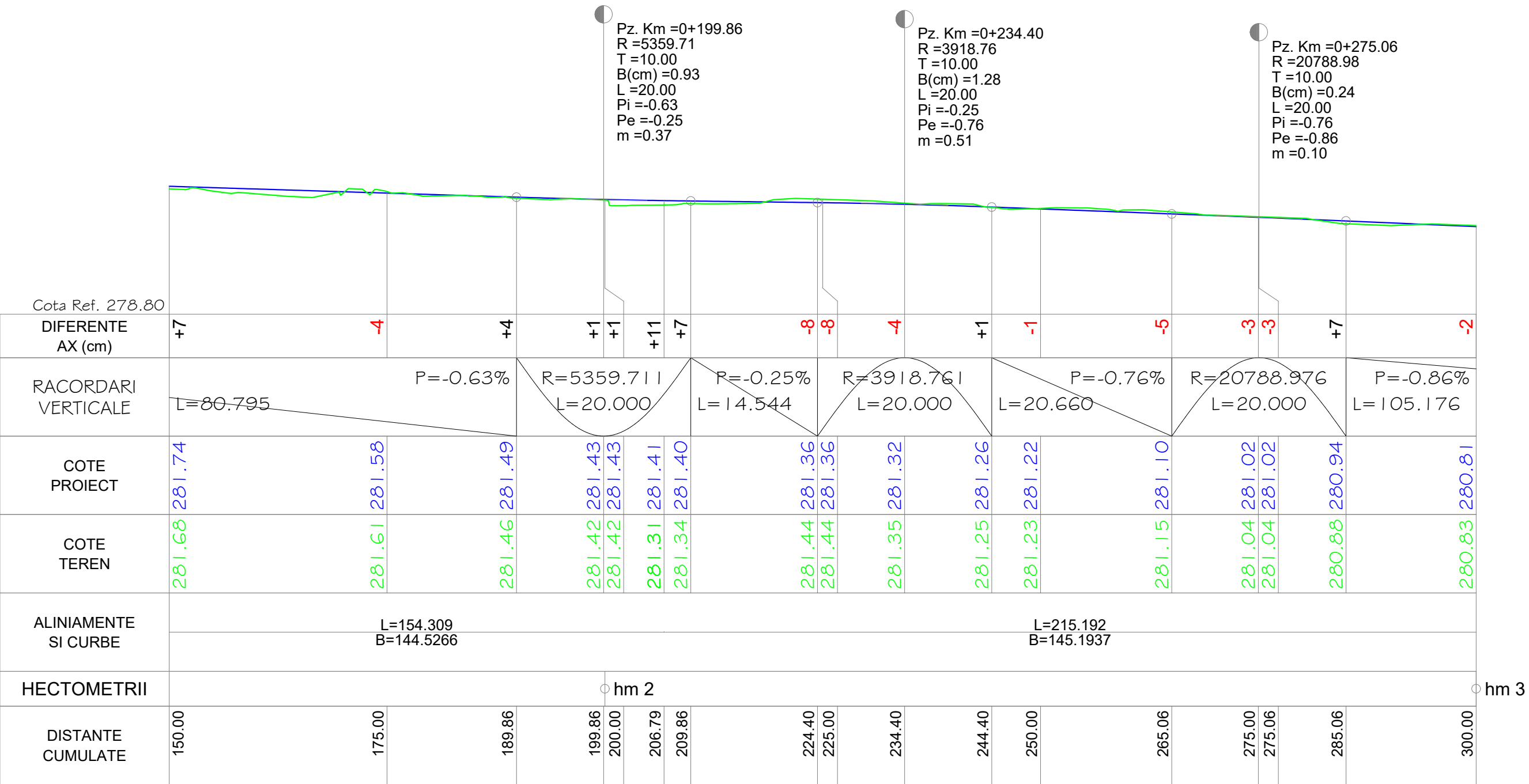
PROFIL LONGITUDINAL Trotuar proiectat DE LA 150.000 LA 300.000 SCARA : ORIZ 1 :500 VERT 1 :100
