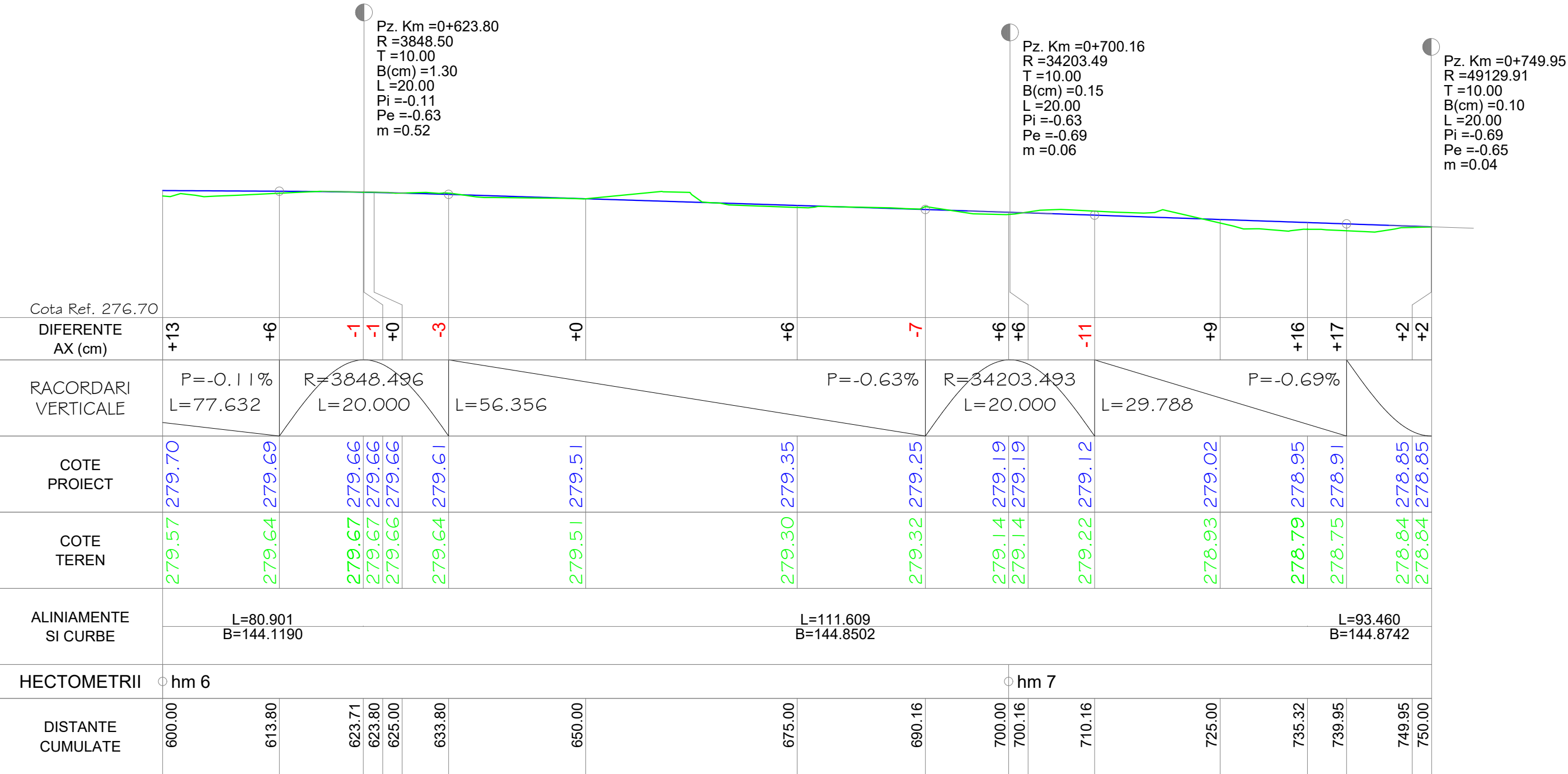
PROFIL LONGITUDINAL Trotuar proiectat DE LA 600.000 LA 750.000 SCARA : ORIZ 1 :500 VERT 1 :100
