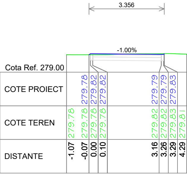
Pz. KM 515.32 Trotuar proiectat
