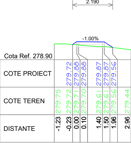
Pz. KM 500.00 Trotuar proiectat
