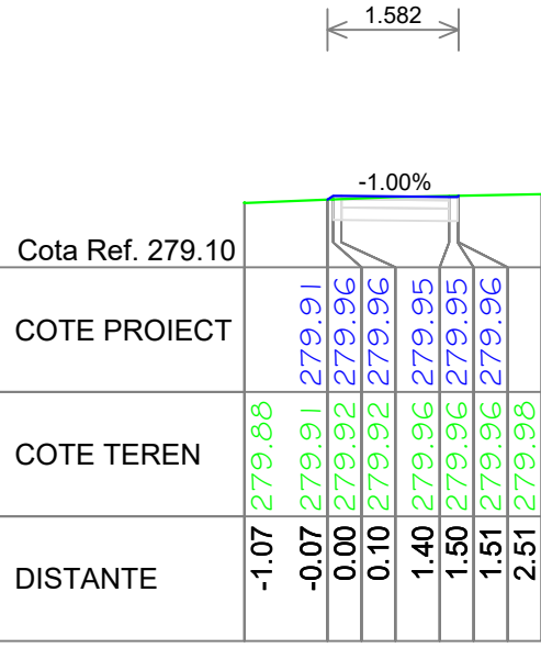
Pz. KM 475.00 Trotuar proiectat
