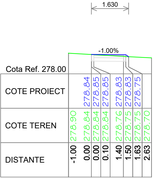
Pz. KM 750.00 Trotuar proiectat
