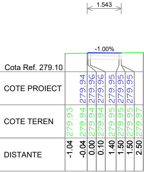
Pz. KM 450.00 Trotuar proiectat
