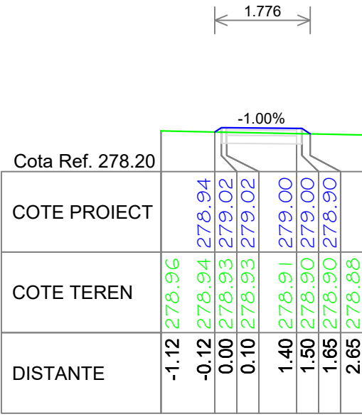
Pz. KM 725.00 Trotuar proiectat
