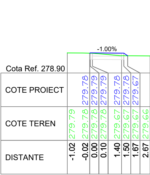
Pz. KM 525.00 Trotuar proiectat
