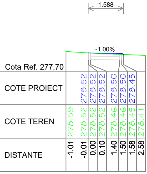
Pz. KM 825.00 Trotuar proiectat
